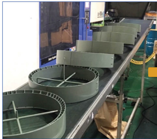
내부압력 보강용(링)
