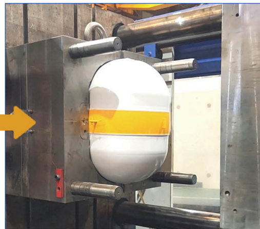
인서트사출(고리)
